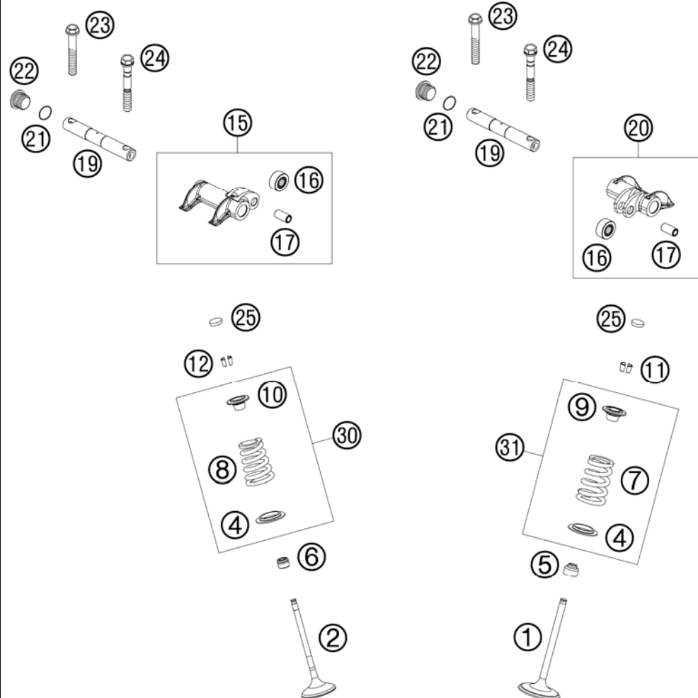
AUSLASS / EXHAUST
