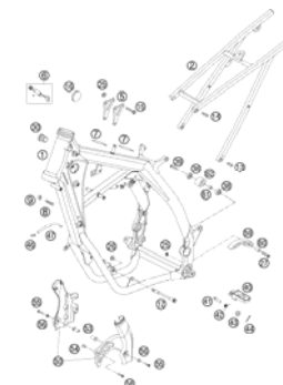
FRAME, SUB FRAME
