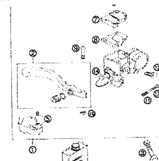
FUSSBREMSBETÄTIGUNG SENIOR LC REAR BRAKE CONTROL SENIOR LC
