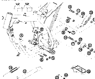
RAHMEN, SEITENSTÄNDER JUNIOR LC FRAME, SIDE STAND JUNIOR LC
