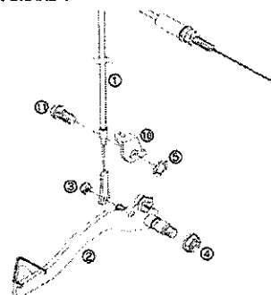
FUSSBREMSBETÄTIGUNG JUNIOR LC REAR BRAKE CONTROL JUNIOR LC
