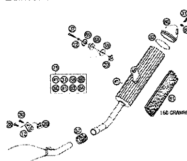
AUSPUFFANLAGE EXHAUST SYSTEM
