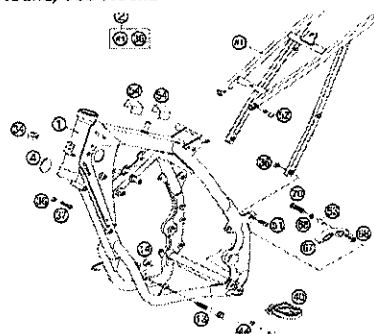
RAHMEN, AUSLEGER FRAME, SUB FRAME
