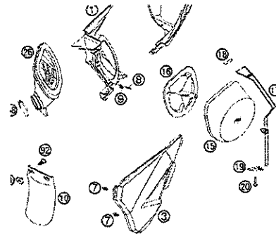
LUFTFILTERKASTEN AIR FILTER BOX
