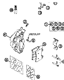
BREMSZANGE VORNE BRAKE CALIPER FRONT
