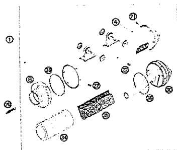
ENDÄMPFER EXHAUST SILENCER
