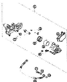
BREMSZANGE HINTEN BRAKE CALIPER REAR
