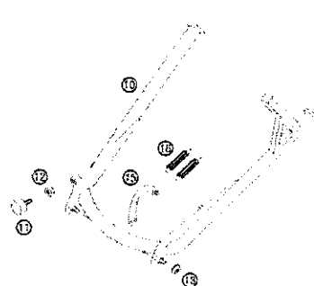
MITTELSTÄNDER CENTER STAND
