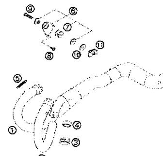
KRÜMMER EXHAUST PIPES
