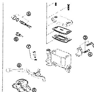
HANDBREMSZYLINDER BREMBO HAND BRAKE CYLINDER BREMBO
