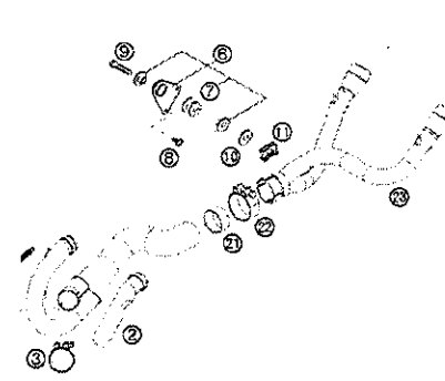
KRÜMMER PIPES
