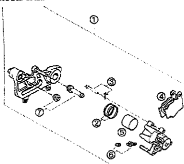
BREMSZANGE HINTEN BREMBO BRAKE CALIPER REAR BREMBO
