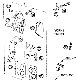
BREMSZANGE VORNE BREMBO BRAKE CALIPER FRONT BREMBO
