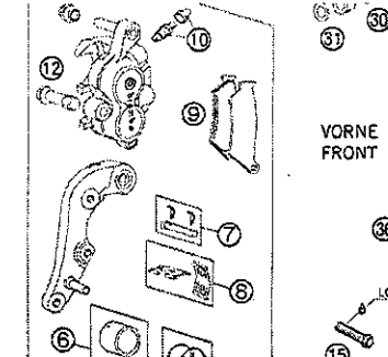
BREMSZANGE VORNE BRAKE CALIPER FRONT
