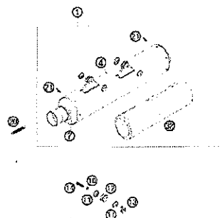
ENDDÄMPFER 450-525 SX EXHAUST SILENCER 450-525 SX
