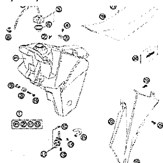
TANK, SITZBANK, VERKLEIDUNG 450-525 SX TANK, SEAT, COVER 450-525 SX
