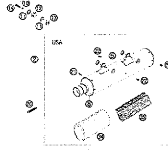
ENDDÄMPFER 250-525 EXC + MXC EXHAUST SILENCER 250-525 EXC + MXC
